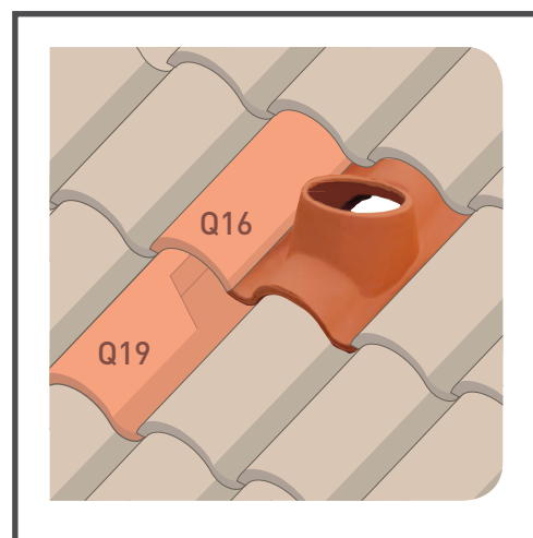
Kit lanterne 160 mm tuile grand sud: incluant Q19, Q47, Q50, Q16 et bande armée.
