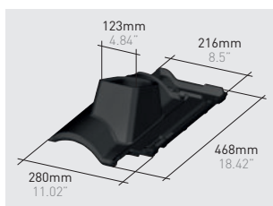
Q132*K | Selectum chimney support klinker
