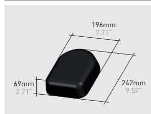
Q135*K | Selectum chimney cover klinker
