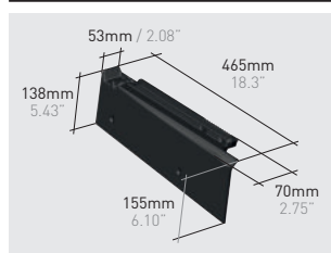
Q133*K | Selectum left side course klinker
