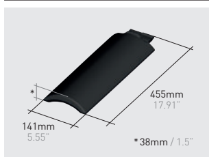
Q130*K | Selectum half roof tile klinker
