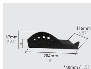
Q136*K | Selectum bird stopper klinker
