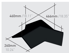
Q111*K | Atica 120° 3 way ridge klinker
