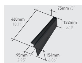
Q116*K | Innova/Vienna right side course klinker
