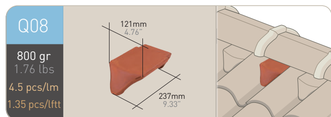
Wedge
