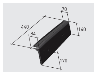
Q88*K | Planum Rive droite klinker
