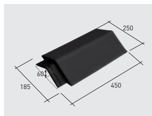
Q90*K | Faîtière Atica 120° klinker
