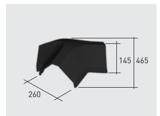
Q146*K | Rencontre 3 directions 45° klinker
