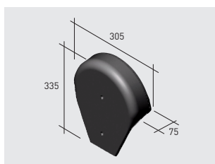
Q83*K | Fronton klinker pour faîtière à pureau variable
