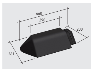
Q109*K | About d'arêtier Atica 120° klinker
