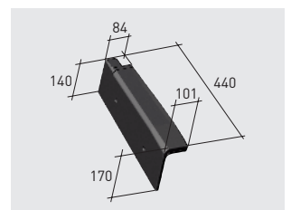
Q89*K | Planum Rive gauche klinker
