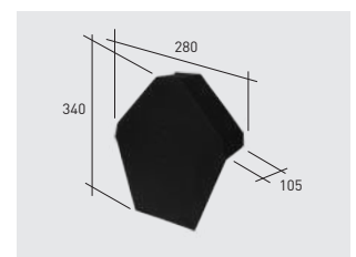
Q147*K | Fronton 45° klinker
