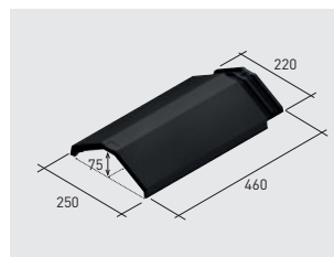
Q120*K | Faîtière Angulaire klinker
