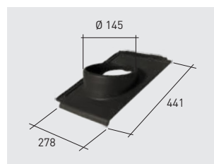
Q87*K | Tuile à douille Planum klinker
