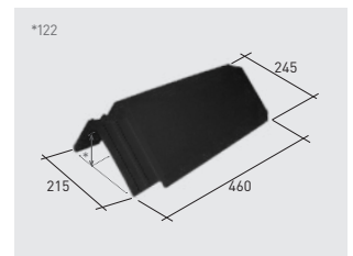
Q145*K | Faîtière 45° klinker
