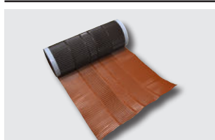
CAM01 / CAMF1 Closoir Aluminium sous Faitage ventilé (souple)
